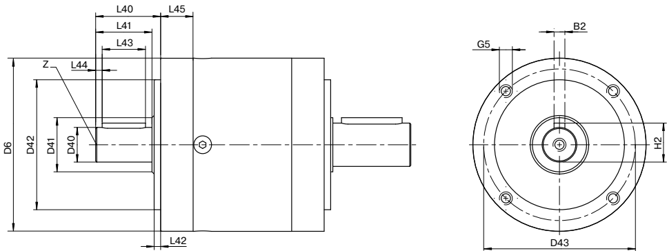
Darstellung entspricht einem PLE080 / 1-stufig / Abtriebswelle mit Passfeder / Antriebswelle – depiction corresponds to a PLE080 / 1-stage / output shaft with feather key / input shaft Alle weiteren Varianten sind im TecDataFinder abrufbar unter www.neugart.com – All other variants can be retrieved in TecDataFinder at www.neugart.com
